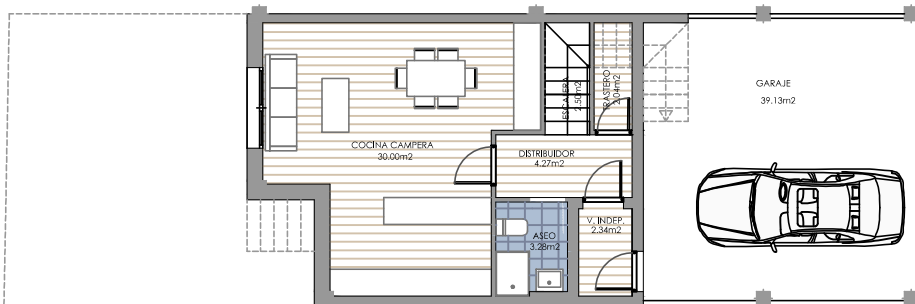
PLANTA SÓTANO
