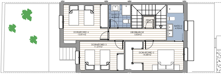
PLANTA PRIMERA
